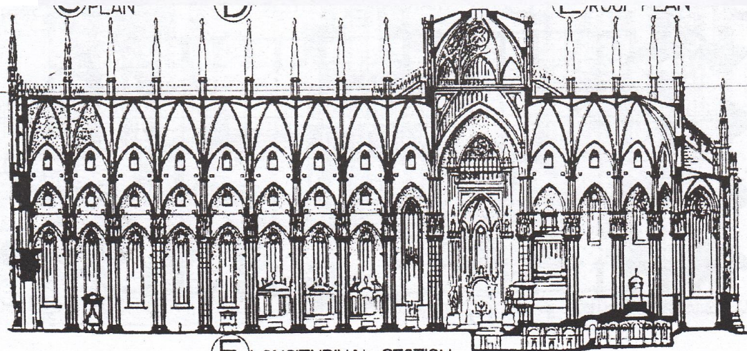
(F) LONGITUDINAL SECTION
