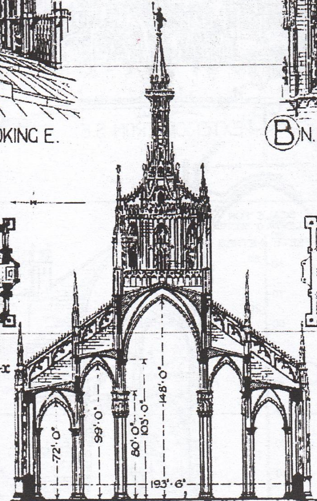
(D) TRANSVERSE SECTION ON x-x
